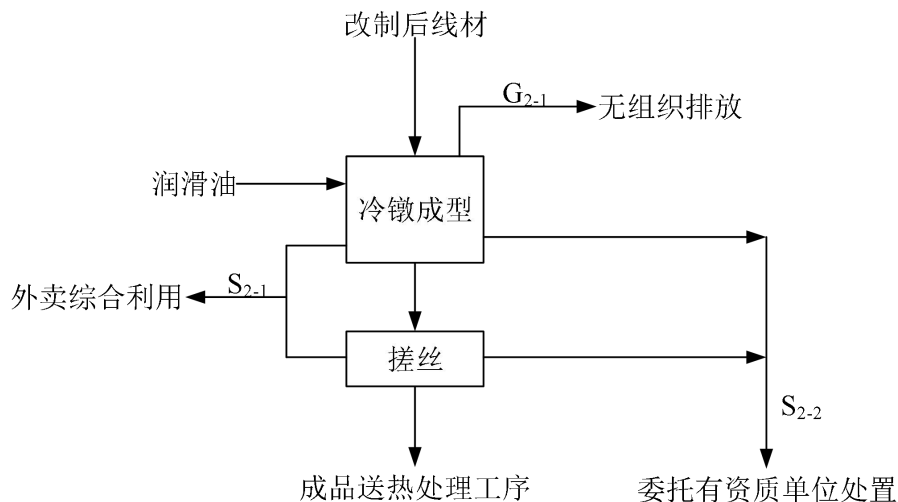
图 3-4 冷成型车间工艺流程图
