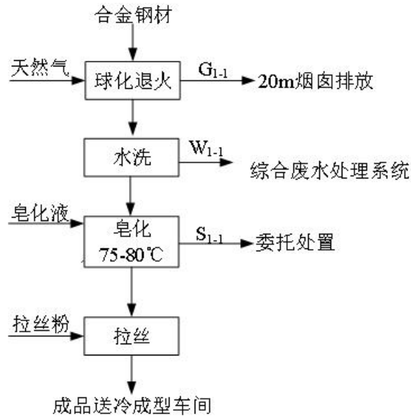
图 3-3 线材改制车间生产工艺流程图
